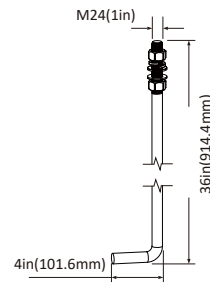
A3 Anchor Bolt
