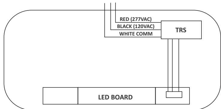
WIRING DAIGRAM
